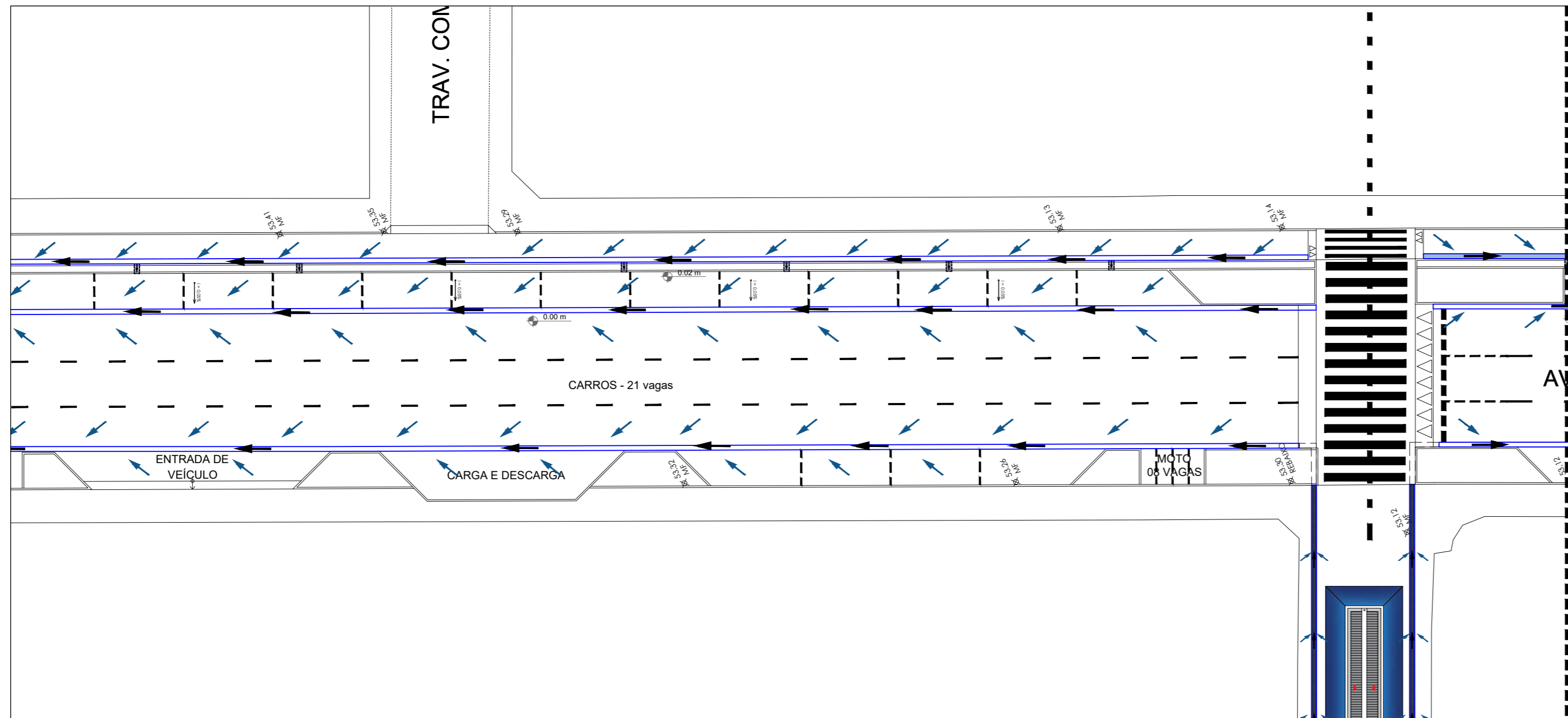
RUA COMANDANTE PETIT - TRECHO 24 escala 1/250
