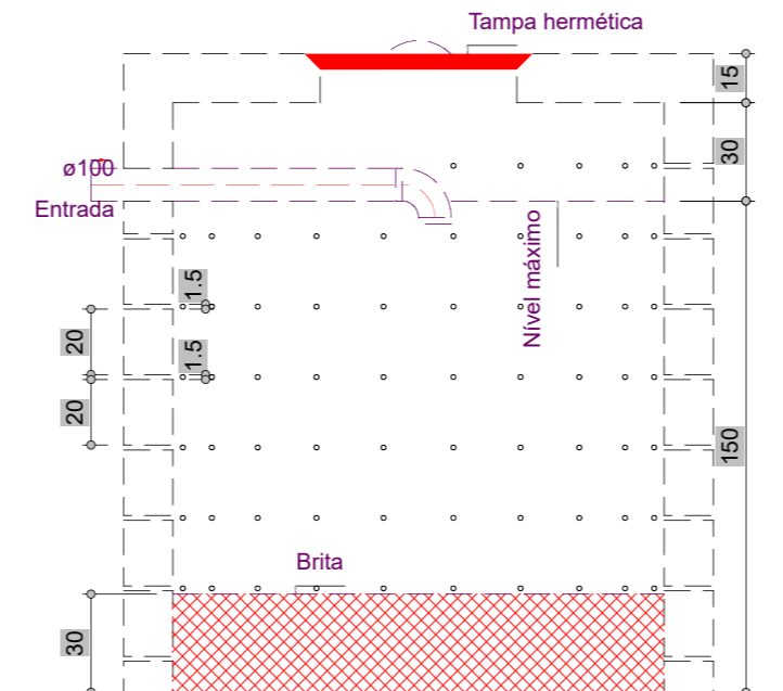
Sumidouro - Pavimento Corte 1 - ESC. 1:25
