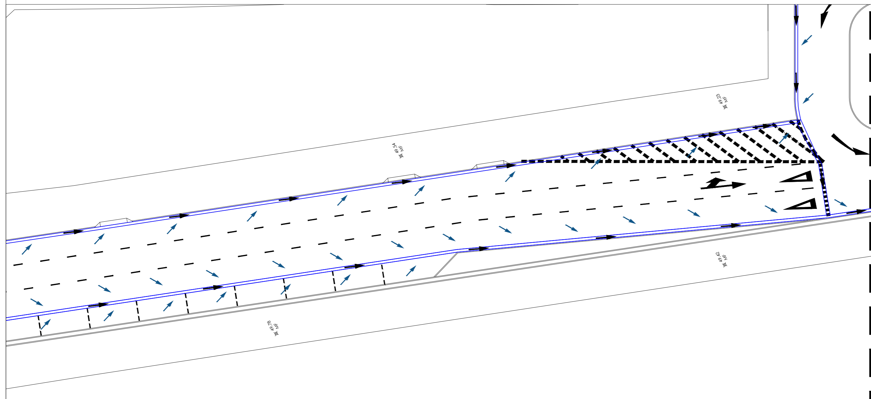
AV. BREVES - TRECHO 13 escala 1/250
