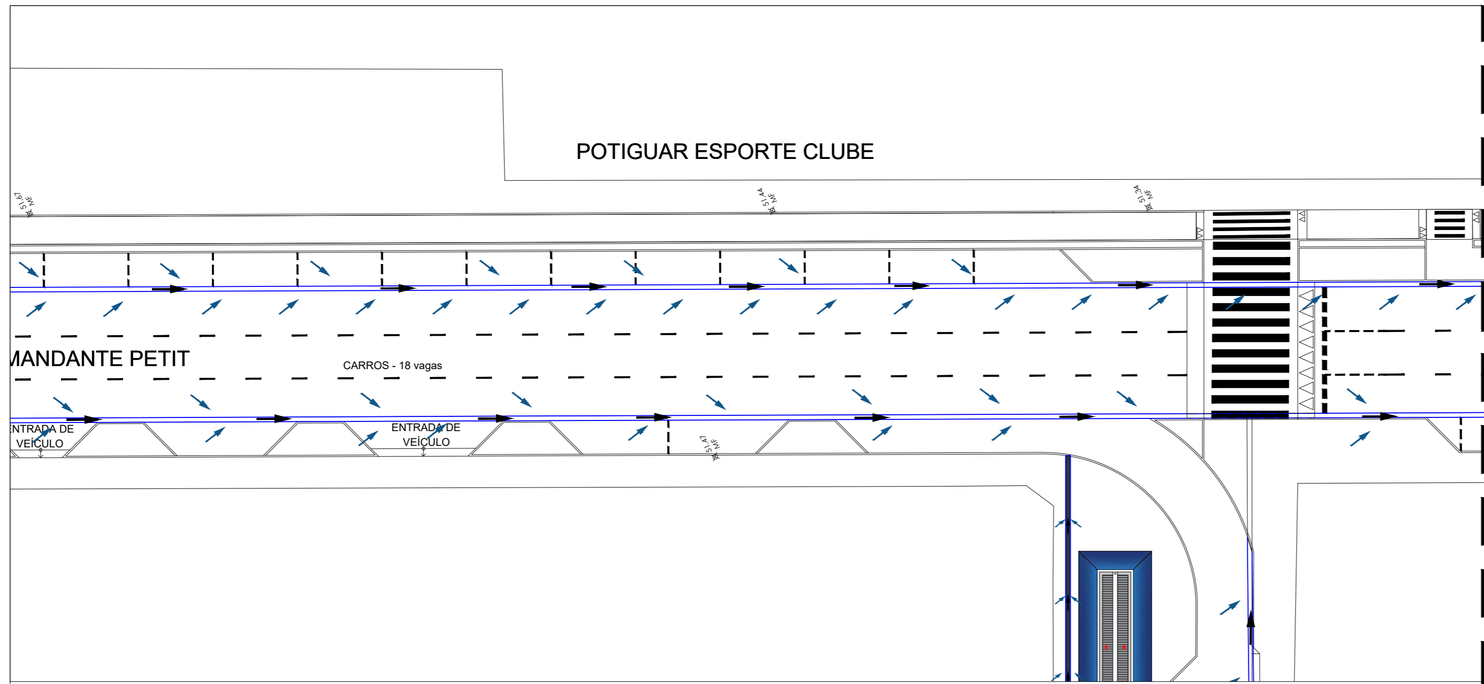
RUA COMANDANTE PETIT - TRECHO 20 escala 1/250
