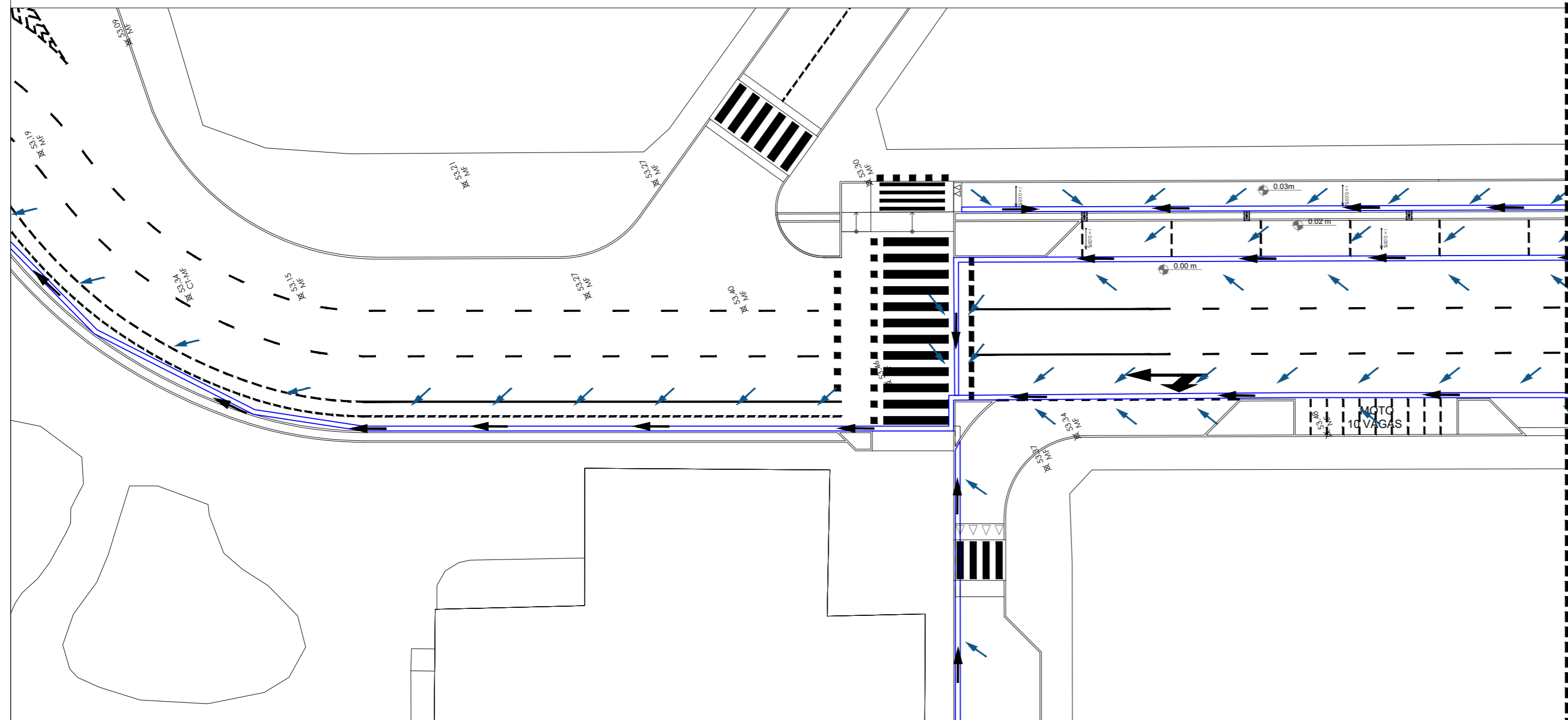
RUA COMANDANTE PETIT - TRECHO 25 escala 1/250
