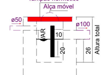
Caixa de gordura - Pavimento Corte 1 - ESC. 1:25
