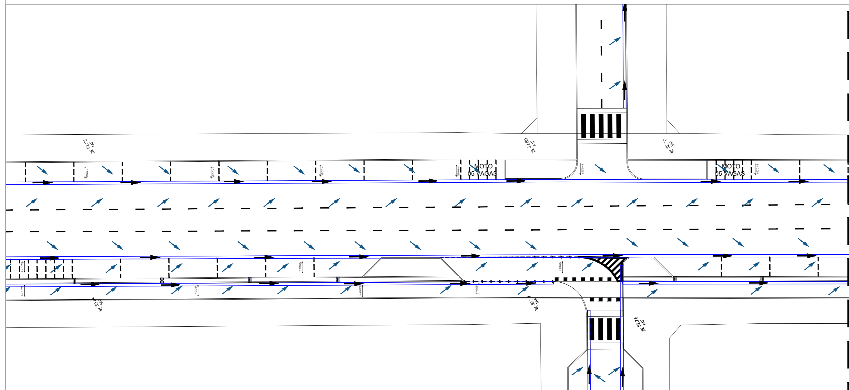
AV. BREVES - TRECHO 08 escala 1/250
