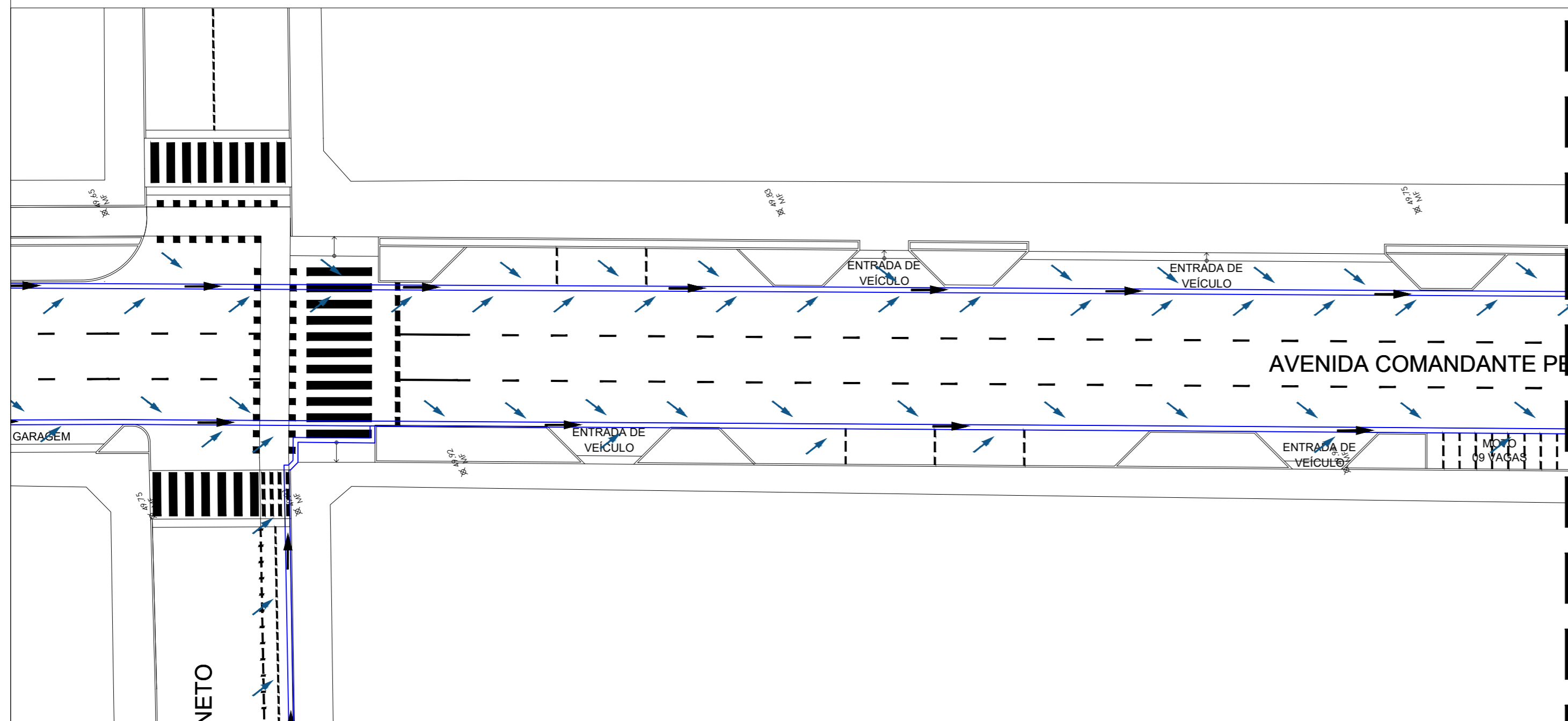
RUA COMANDANTE PETIT - TRECHO 15 escala 1/250
