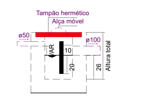
Caixa de gordura - Pavimento Corte 1 - ESC. 1:25
