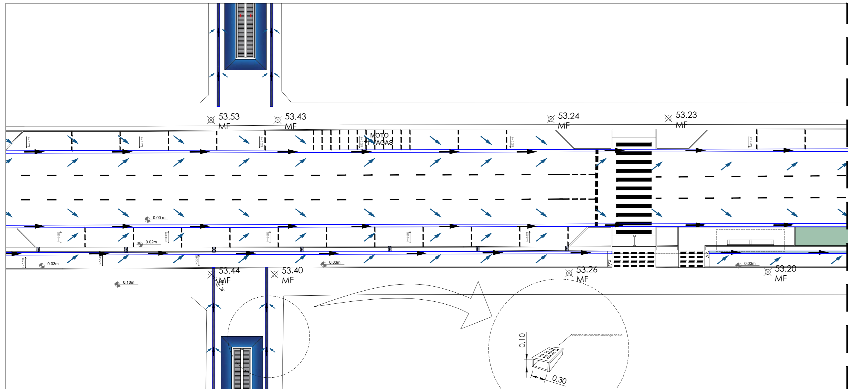
AV. BREVES - TRECHO 05 escala 1/250
