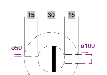
Caixa de gordura - Pavimento Planta baixa - ESC. 1:25
