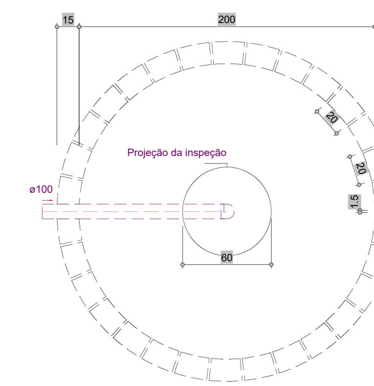
Sumidouro - Pavimento Planta baixa - ESC. 1:25
