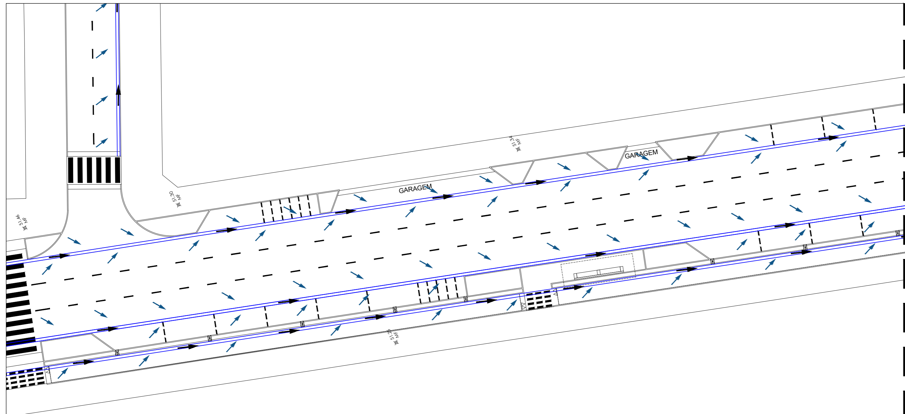
AV. BREVES - TRECHO 12 escala 1/250
