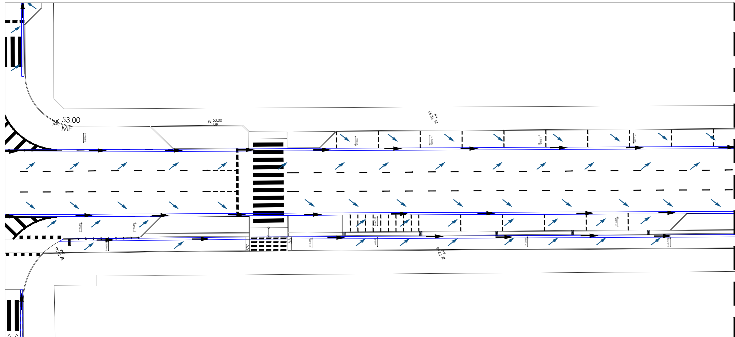
AV. BREVES - TRECHO 07 escala 1/250
