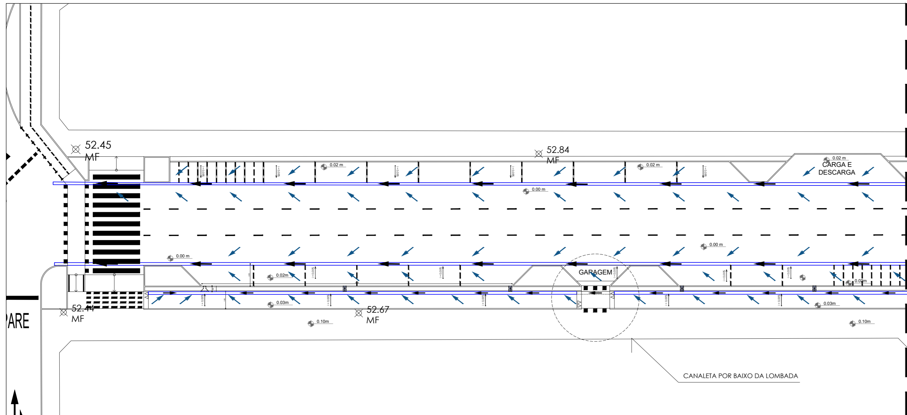
AV. BREVES - TRECHO 01 escala 1/250
