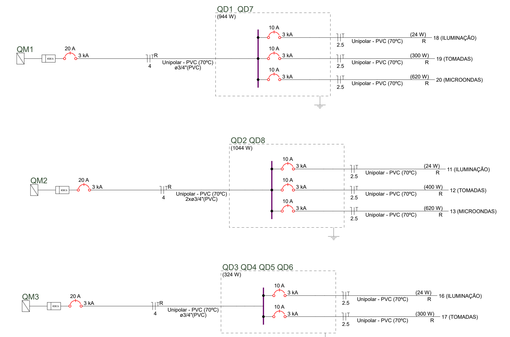
Detalhe ELE-1 Escala 1:25
