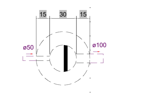
Caixa de gordura - Pavimento Planta baixa - ESC. 1:25
