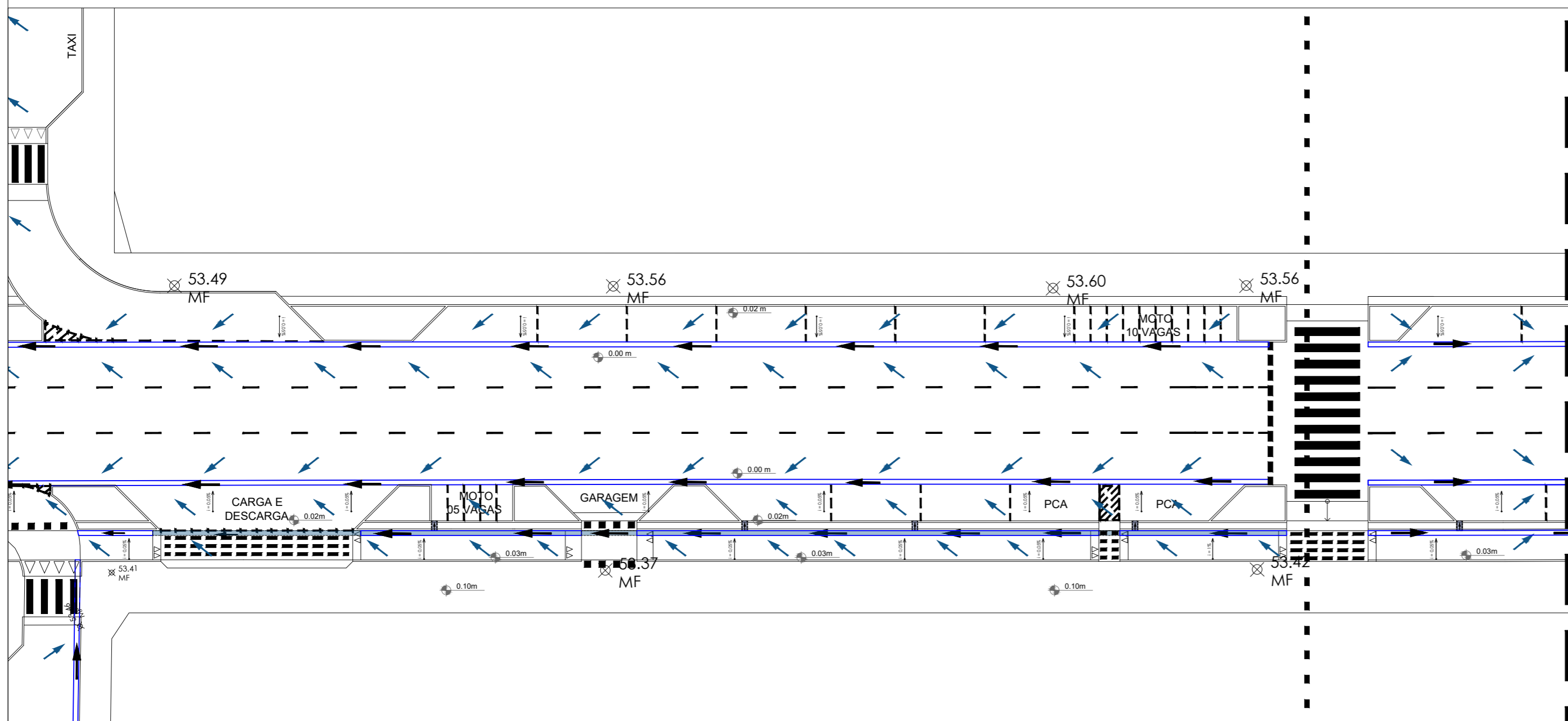
AV. BREVES - TRECHO 04 escala 1/250
