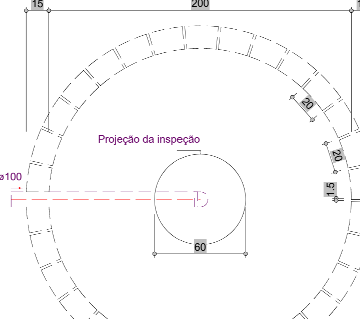
Sumidouro - Pavimento Planta baixa - ESC. 1:25
