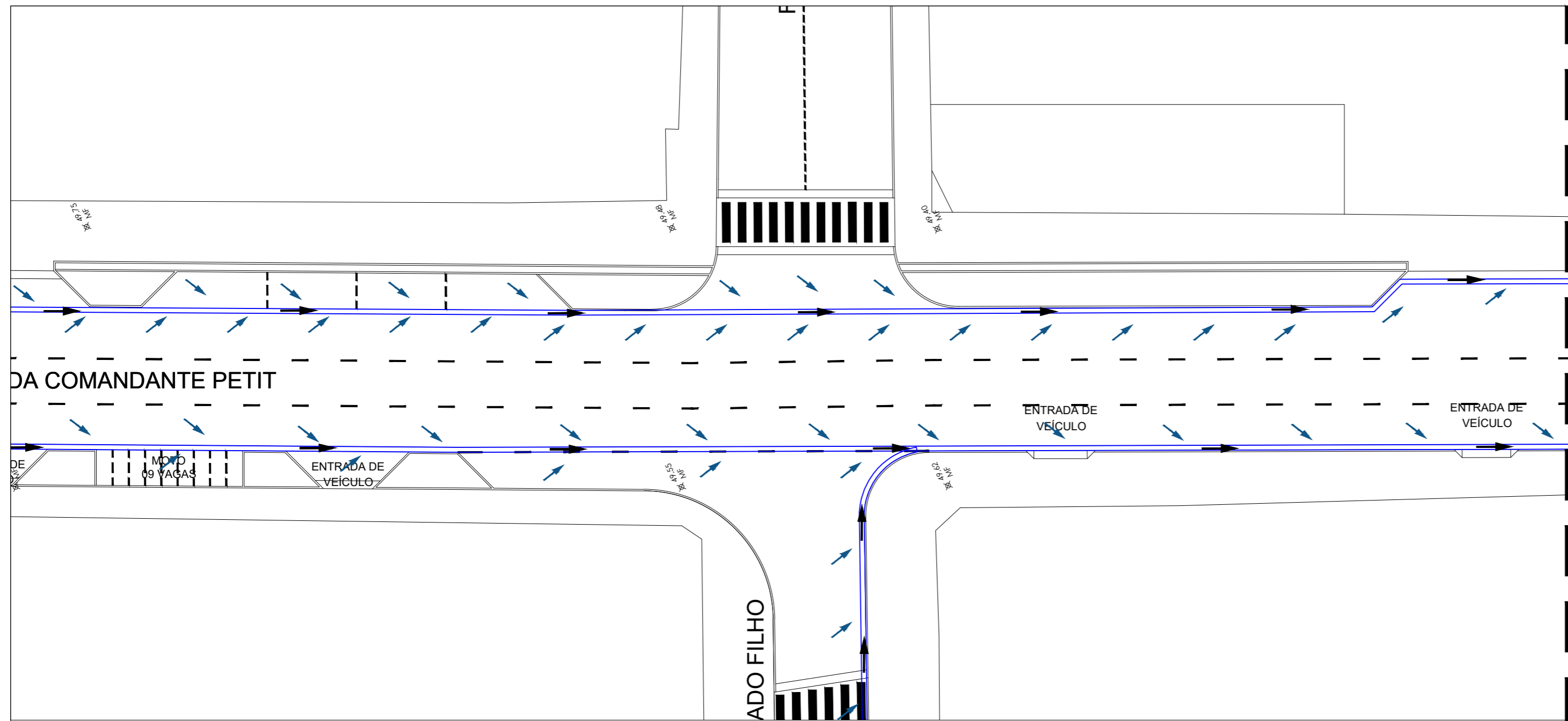
RUA COMANDANTE PETIT - TRECHO 14 escala 1/250
