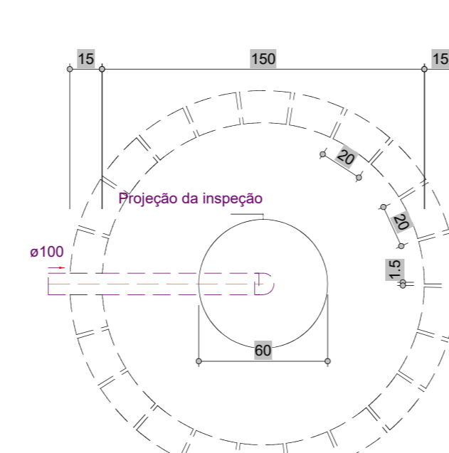
Sumidouro - Pavimento Planta baixa - ESC. 1:25
