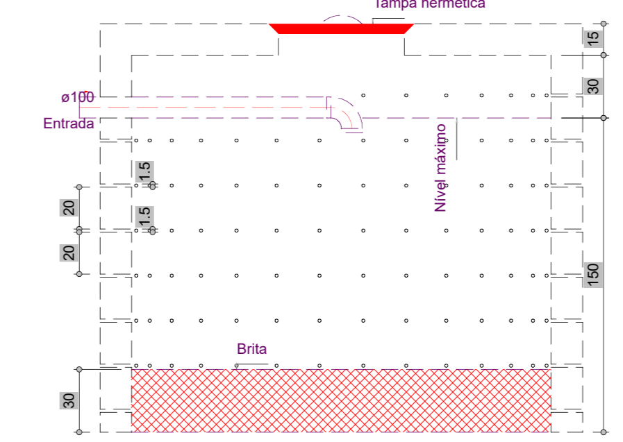
Sumidouro - Pavimento Corte 1 - ESC. 1:25
