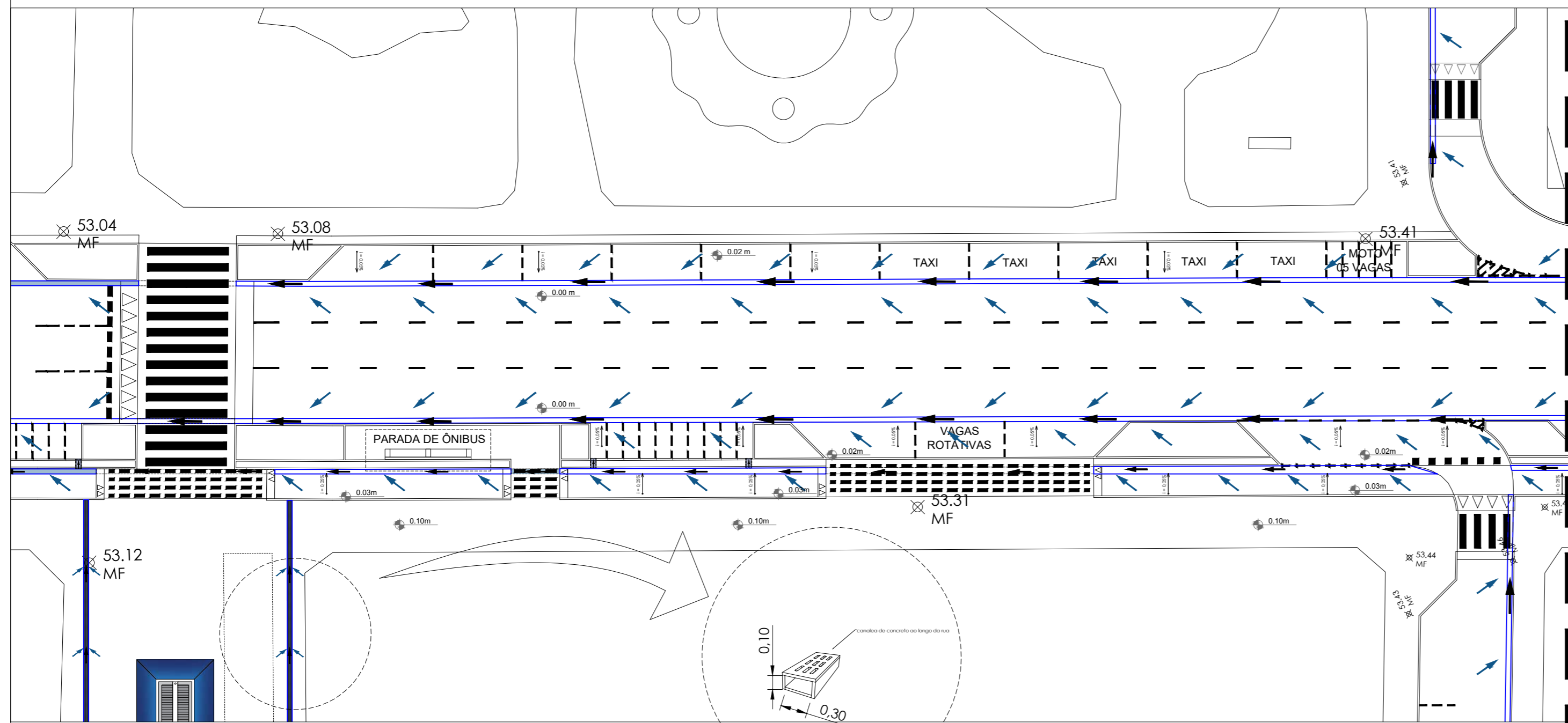
AV. BREVES - TRECHO 02 escala 1/250
