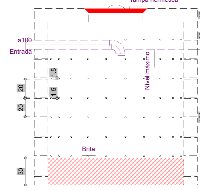
Sumidouro - Pavimento Corte 1 - ESC. 1:25
