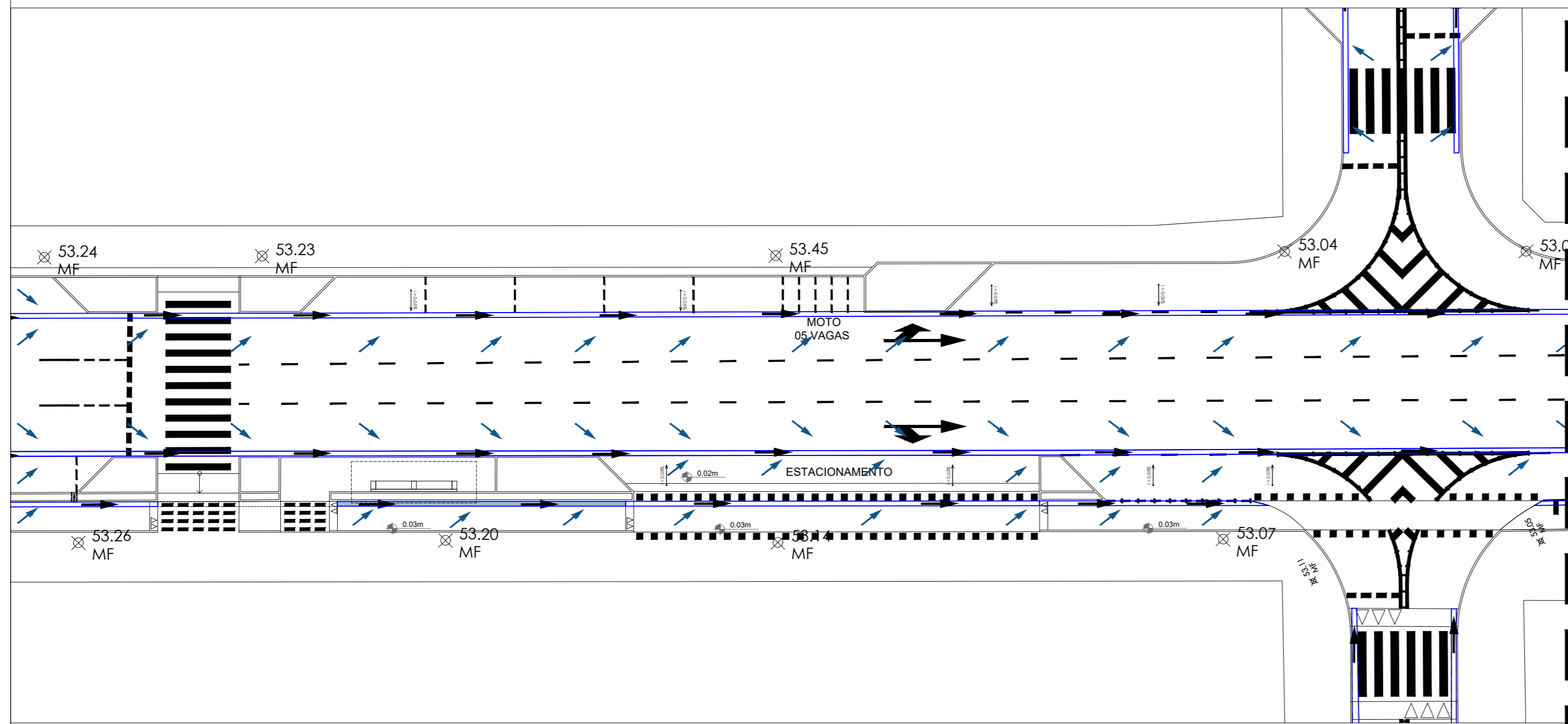
AV. BREVES - TRECHO 06 escala 1/250
