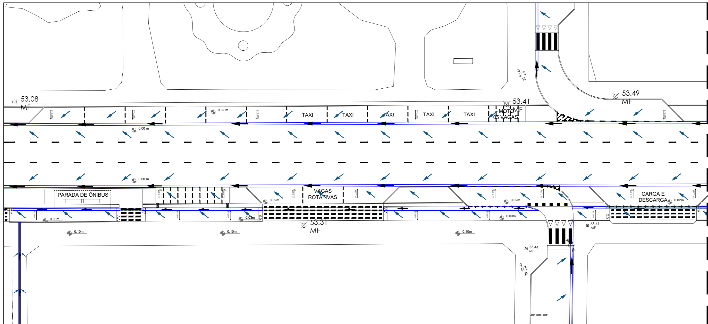
AV. BREVES - TRECHO 03 escala 1/250
