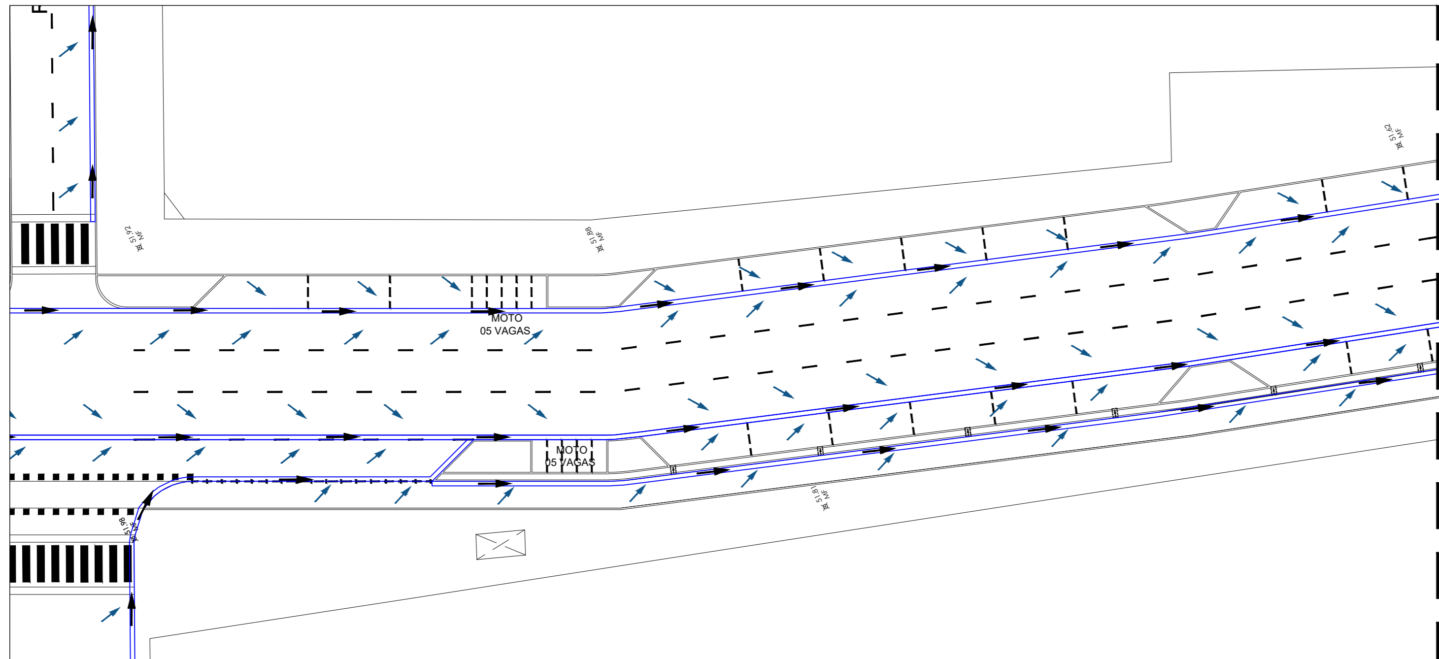
AV. BREVES - TRECHO 10 escala 1/250
