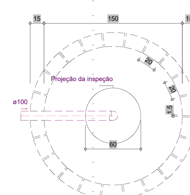
Sumidouro - Pavimento Planta baixa - ESC. 1:25
