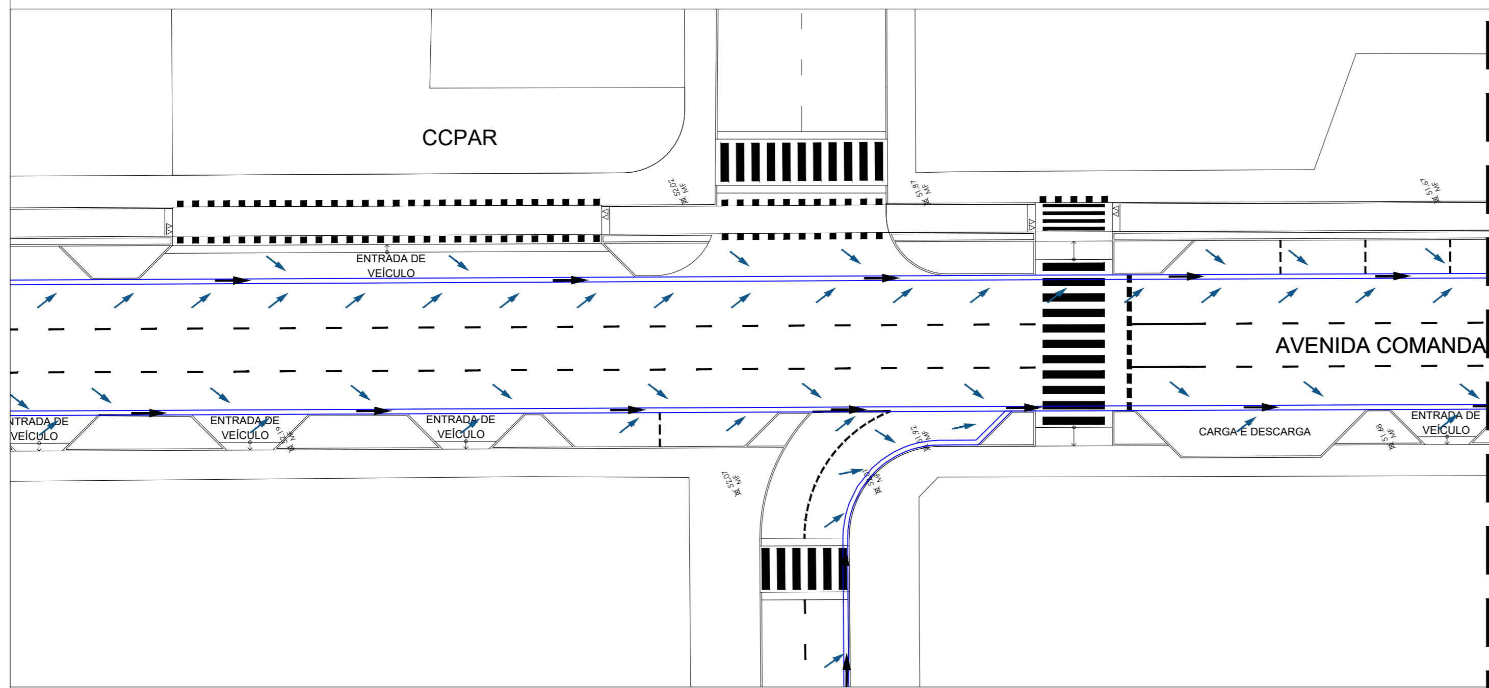
RUA COMANDANTE PETIT - TRECHO 21 escala 1/250
