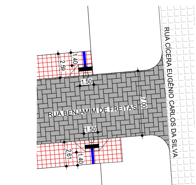
13 DETALHE - CRUZAMENTO RUA BENJAMIM DE FREITAS COM RUA CÍCERA EUGÊNIO CARLOS DA SILVA ESCALA:1/250
