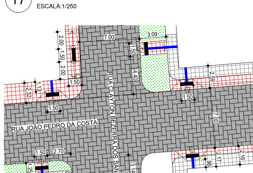
20 DETALHE - CRUZAMENTO RUA JOÃO PEDRO DA COSTA COM RUA CLAYTON BEZERRA DOS SANTOS ESCALA:1/250
