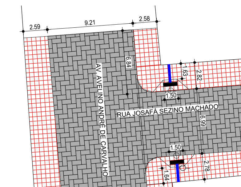
16 DETALHE - CRUZAMENTO RUA JOSAFÁ SEZINO MACHADO COM AV. AVELINO ANDRÉ DE CARVALHO ESCALA:1/250
