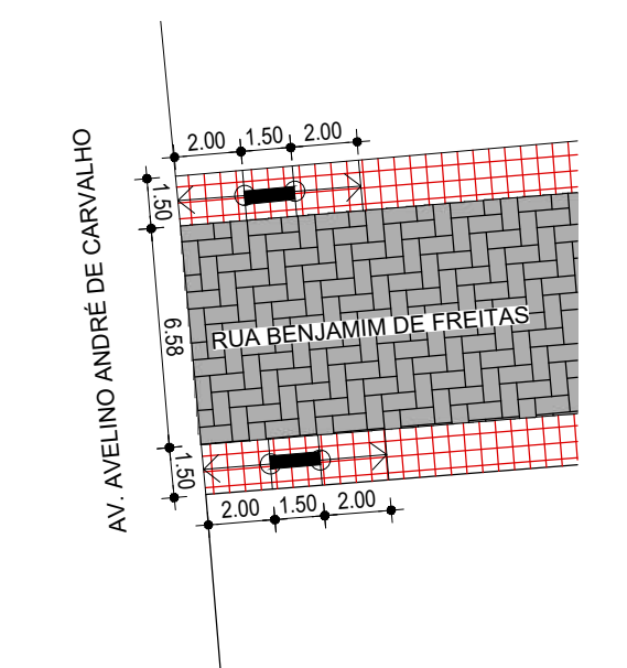
11 DETALHE - CRUZAMENTO RUA BENJAMIM DE FREITAS COM AV. AVELINO ANDRÉ DE CARVALHO ESCALA:1/250
