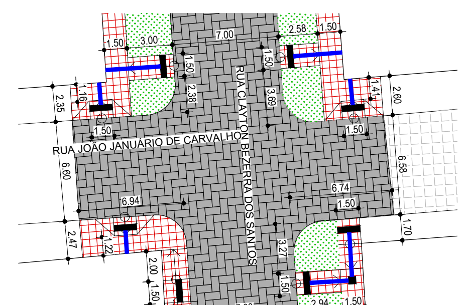
15 DETALHE - CRUZAMENTO RUA JOÃO JANUÁRIO DE CARVALHO COM RUA CLAYTON BEZERRA DOS SANTOS ESCALA:1/250
