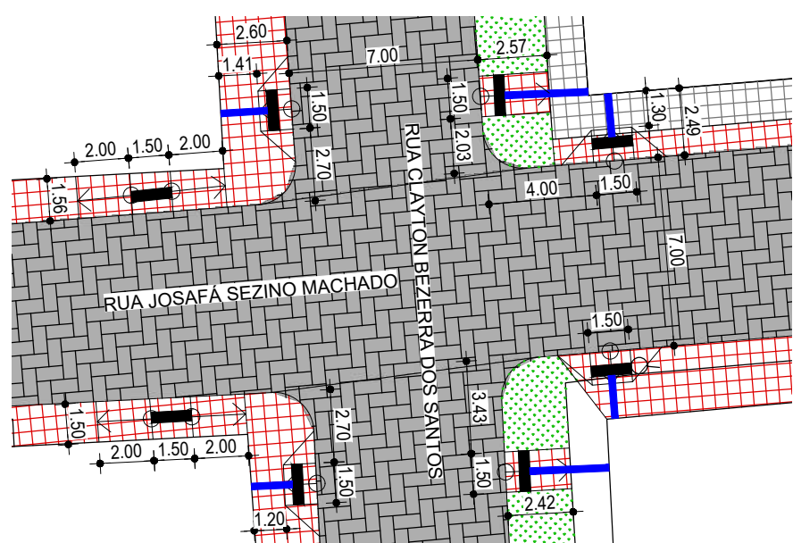
17 DETALHE - CRUZAMENTO RUA JOSAFÁ SEZINO MACHADO COM RUA CLAYTON BEZERRA DOS SANTOS ESCALA:1/250
