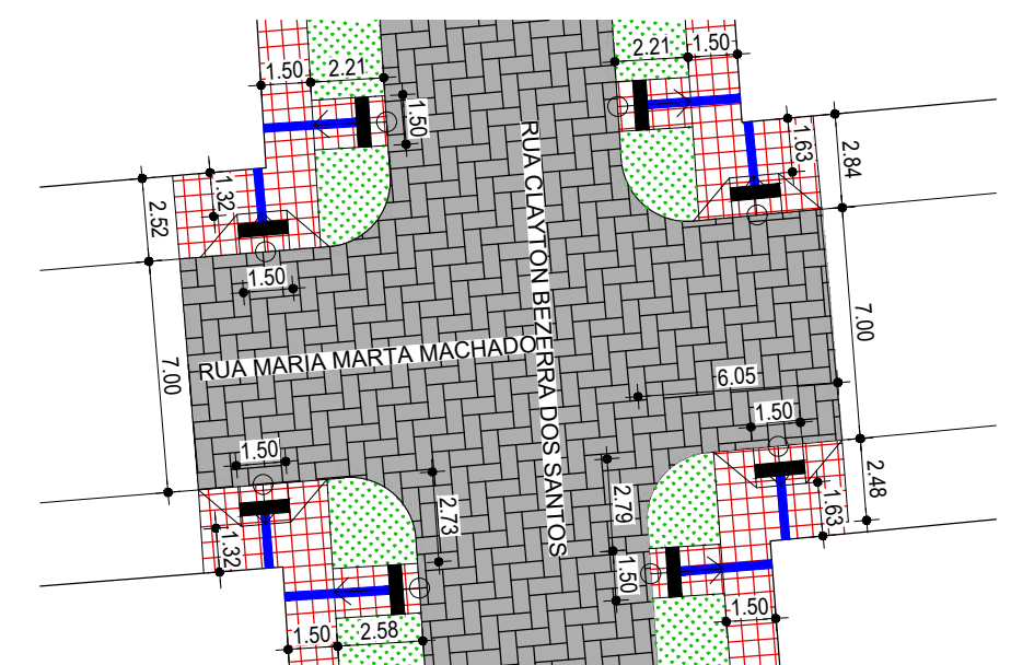
14 DETALHE - CRUZAMENTO RUA MARIA MARTA MACHADO COM RUA CLAYTON BEZERRA DOS SANTOS ESCALA:1/250
