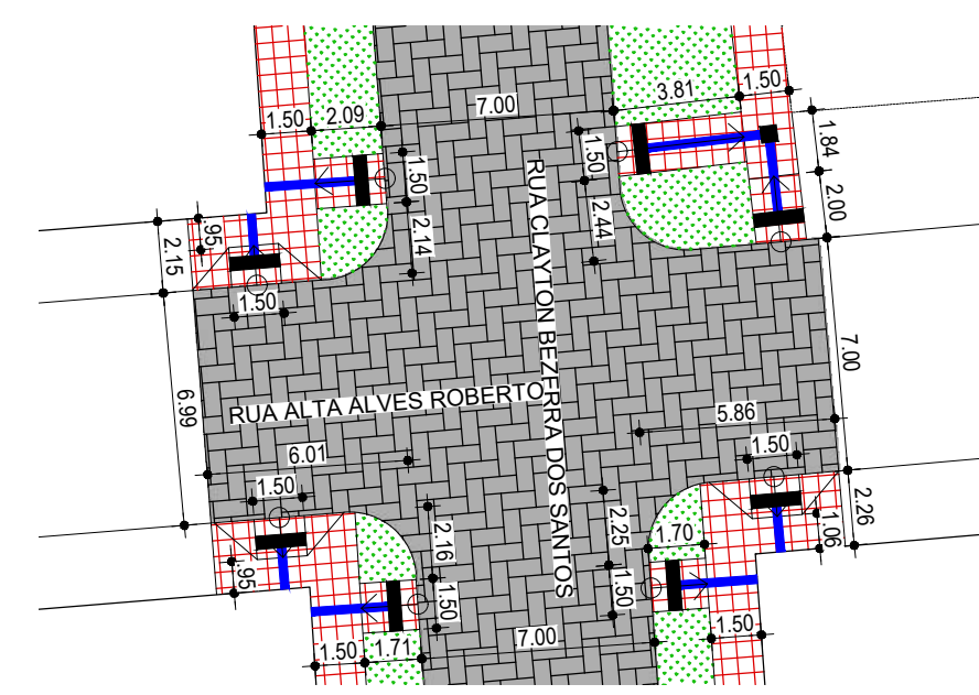
10 DETALHE - CRUZAMENTO RUA ALTA ALVES ROBERTO COM RUA CLAYTON BEZERRA DOS SANTOS ESCALA:1/250
