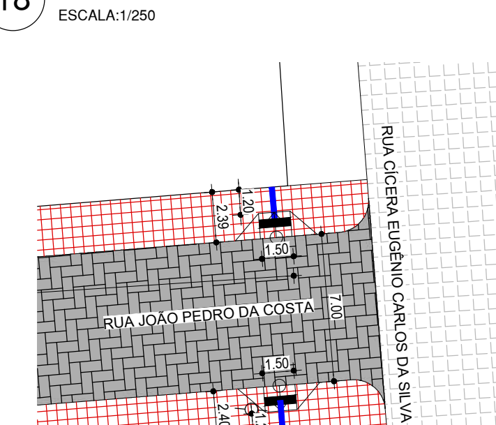
21 DETALHE - CRUZAMENTO RUA JOÃO PEDRO DA COSTA COM RUA CÍCERA EUGÊNIO C. DA SILVA ESCALA:1/250
