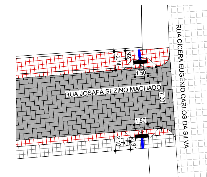
18 DETALHE - CRUZAMENTO RUA JOSAFÁ SEZINO MACHADO COM RUA CÍCERA EUGÊNIO C. DA SILVA ESCALA:1/250
