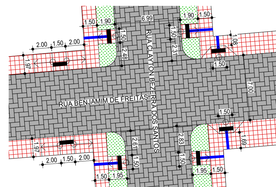
12 DETALHE - CRUZAMENTO RUA BENJAMIM DE FREITAS COM RUA CLAYTON BEZERRA DOS SANTOS ESCALA:1/250
