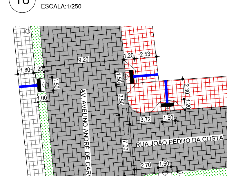
19 DETALHE - CRUZAMENTO RUA JOÃO PEDRO DA COSTA COM AV. AVELINO ANDRÉ DE CARVALHO ESCALA:1/250
